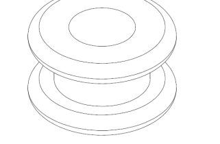
854195 RUBBER GROM- MET .281 ID X .625 OD
