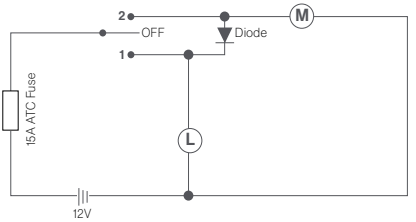
Diagrama de cableado
