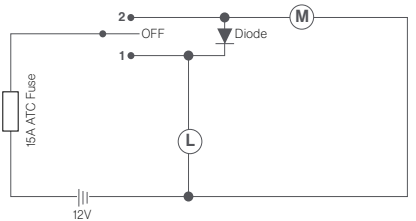
Schéma de câblage
