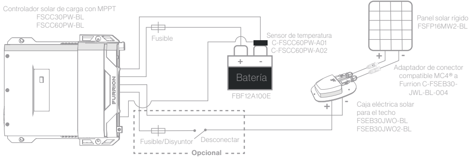
Diagrama del sistema de conexiones
