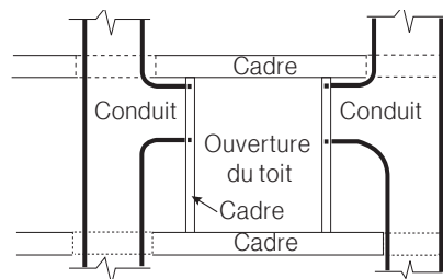
VUE DE DESSUS (ARRIÈRE DU AUTO-CARAVANE)
