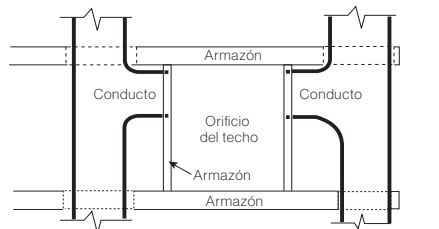
VISTA SUPERIOR (PARTE TRASERA DEL RV)
