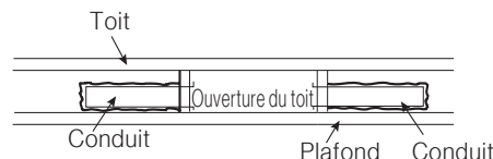
VUE LATÉRALE (VERS L'ARRIÈRE DE L'AUTO-CARAVANE)
