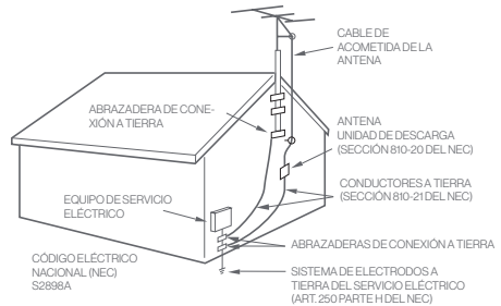
EJEMPLO DE CONEXIÓN A TIERRA DE LA ANTENA SEGÚN EL CÓDIGO ELÉCTRICO NACIONAL
