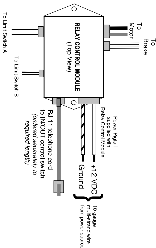
WIRING DIAGRAM:
