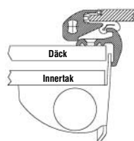
Rullgardin – mått
