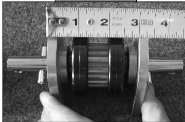
Fig. 6 - Gear Pack
