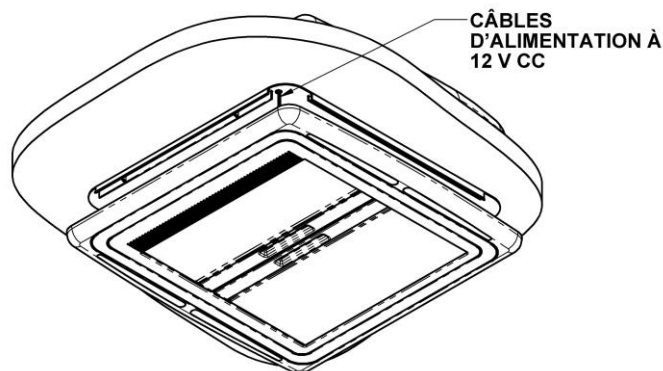
LANTERNEAU ÉCLAIRÉ
