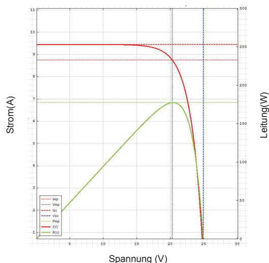
RNG-175DB-H Eigenschaften gegen Spannung
