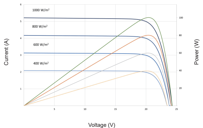
RSP100D-BK Die Eigenschaften gegenüber der Spannung
