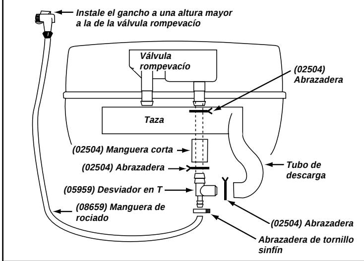
Figura 1 - Vista trasera
