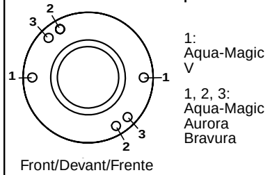
Fig. 2 Bolt Pattern/schema des boulons/ Distribución de los pernos
