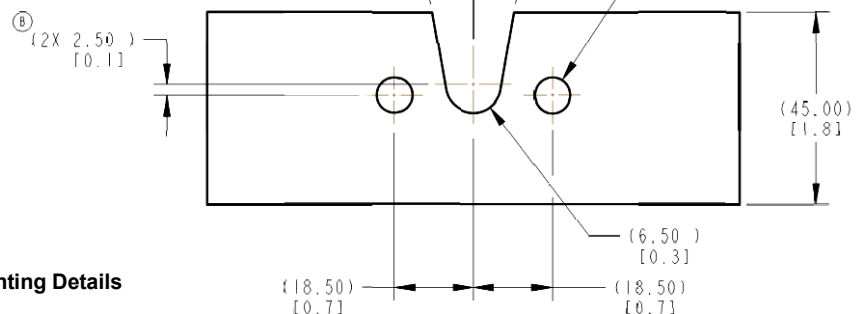
CUTOUT
