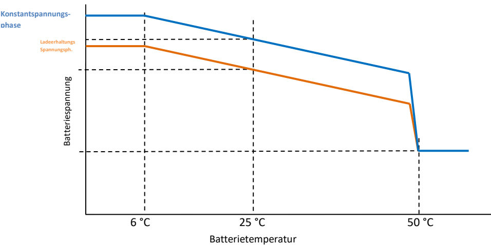
Abbildung 1: Temperaturkompensationskurve
