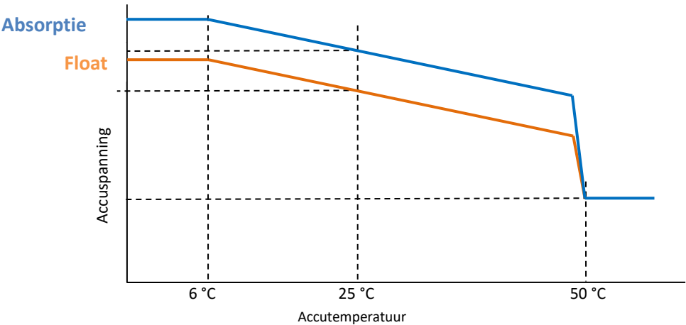
Afbeelding 1: temperatuurcompensatiecurve
